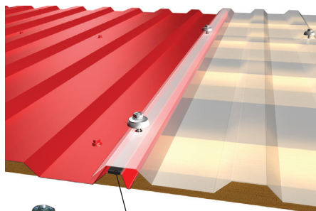
Саморез 4.8 х 50 с термошайбой
